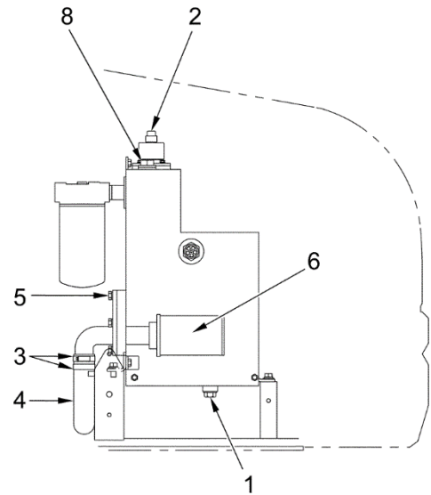
Posición de descarga del aceite hidráulico
