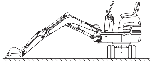
Posición de descarga del aceite hidráulico
