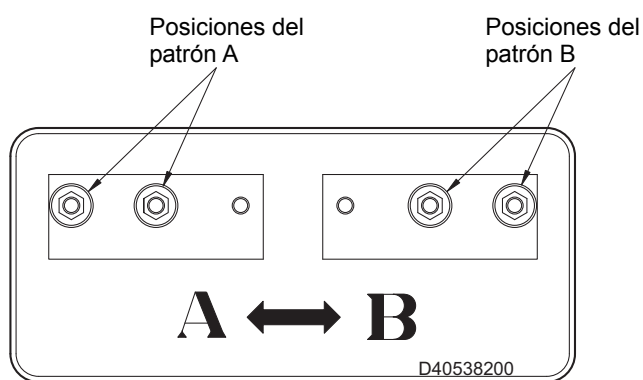
Placa de cambio del sistema de funcionamiento
